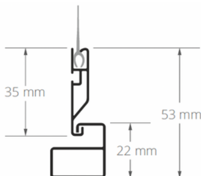
Wysokość listwy dolnej i listwy hakowej.
