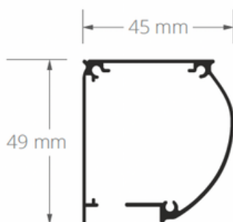
Wymiary kasety.
